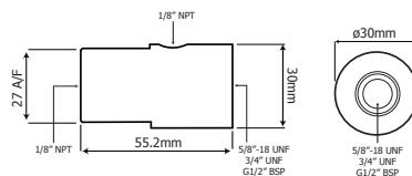
Cella portasonda opzionale (vedere accessori e spare)
